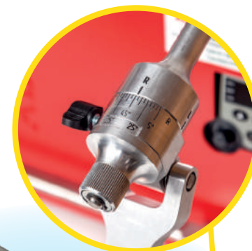
Манипулятор с функцией выставления угла
